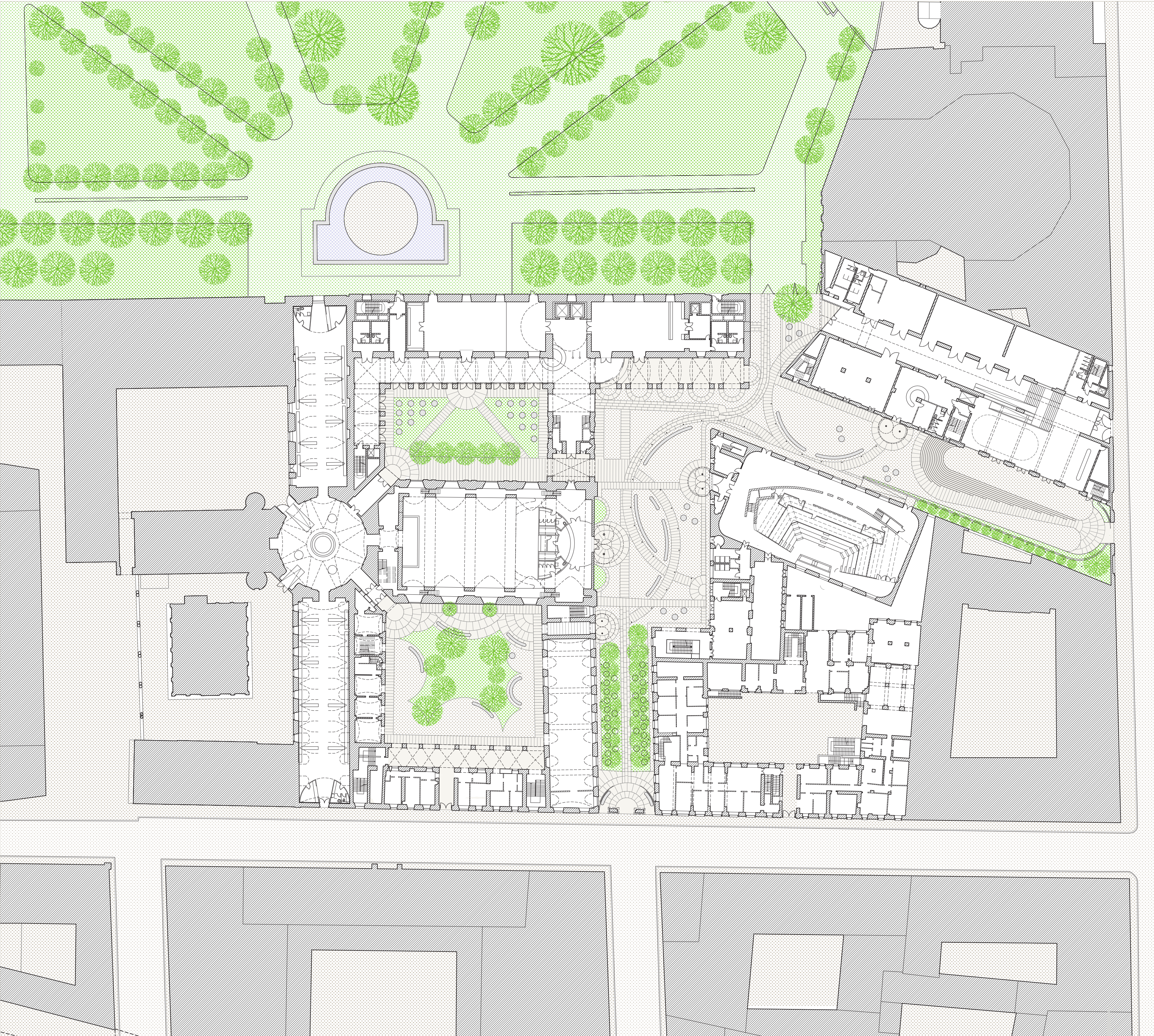
La nuova Cavallerizza Reale, planimetria generale scala 1:500
